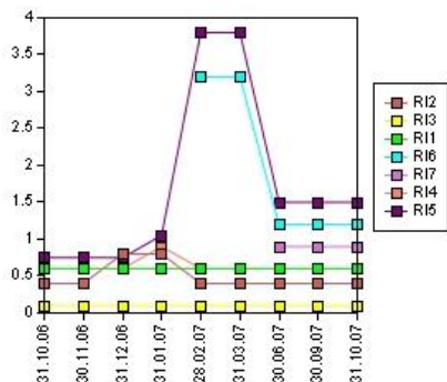
Abb.02: Risikotrendanalyse
