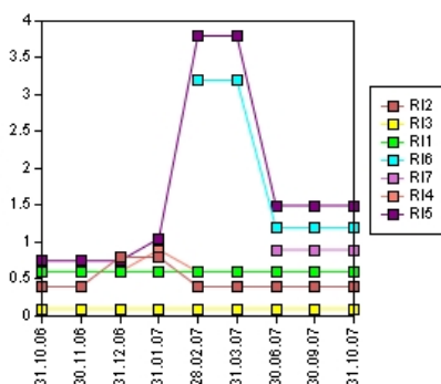
Abb.02: Risikotrendanalyse
